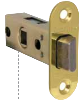
LH 220-45-20 PB латунь
